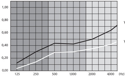
Schallabsorptionsgrad \alpha_{\text{Sabine}}
